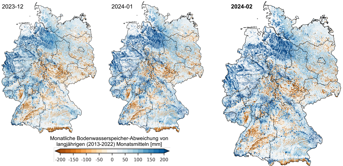
Abb. 1: Monatliche Gesamtspeicherabweichung der vergangenen Jahreszeit mit Bezug auf die langfristigen Monatsmittel von 2013 bis 2022 in mm Wassersäule. Im Falle des eWRB umfasst der Gesamt-Bodenwasserspeicher den flachen Boden bis in tiefere Grundwasserkörper bis 60m Tiefe . Daten: Hindcasts von ParFlow/CLM Simulationen, angetrieben mit ECMWF HRES.
