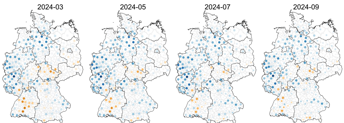
Abb. 3: Saisonale Vorhersagen (2024-Mär bis 2024-Sept) ; Mittel der Anomalien des gesamten Bodenwasserspeichers, ParFlow/CLM Simulationen (initialisiert: 2024-03-01) mit ECMWF SEAS Antrieb (50 Ensemble Member). Punkte: NUTS-3 Verwaltungsebene; Punktgröße: Proportional der Anzahl der Member mit identischem Vorzeichen (positive oder negative Anomalie).
